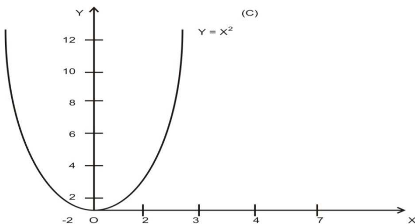
Quadrat Function (द्विघाती फलन)
