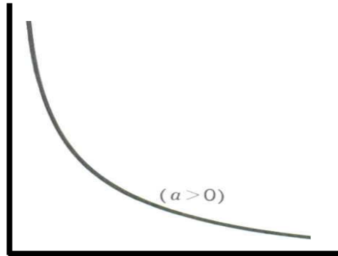
चित्र संख्या 5— अति परवलय लंघन
