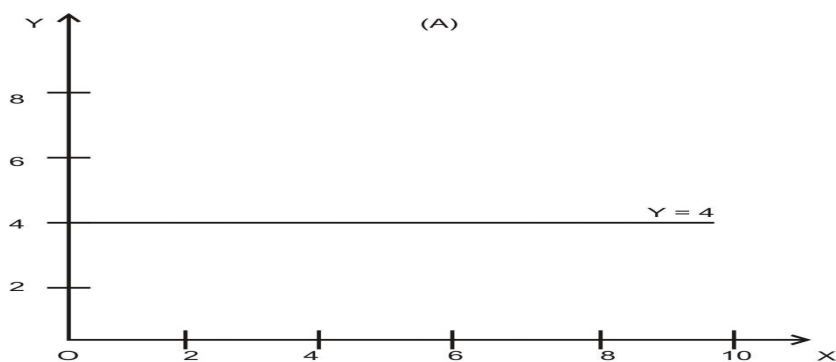
स्थिर फलन Constant function
