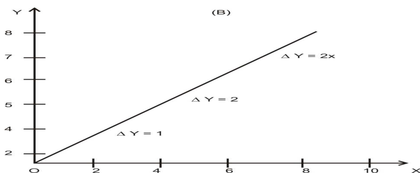
Linear Function (रेखीय फलन)
