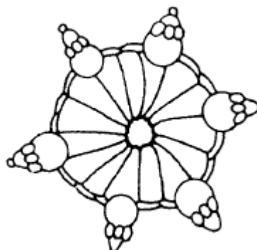
Fig.1.8: Amyllum star
