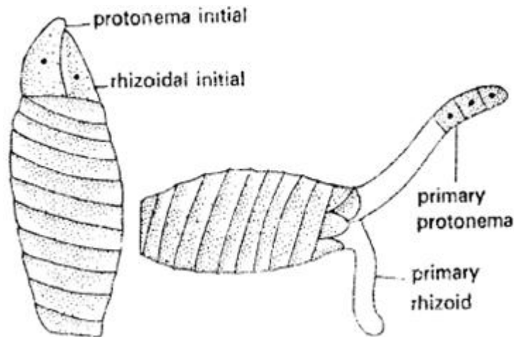
Fig.1.9: Protonema
