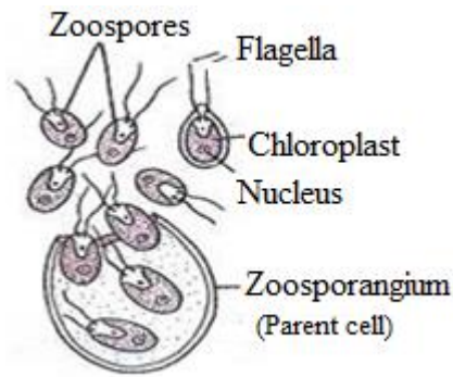
Fig 1.10 A: Zoospores
