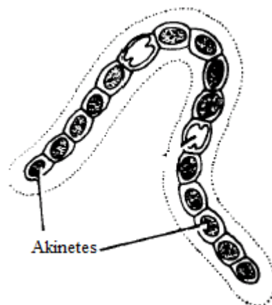
Fig.1.15: Akinete
