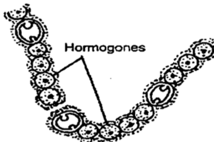
Fig.1.7: Hormogones
